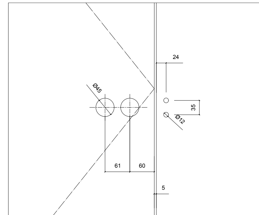
Kombinacija brava + kraća kontra brava za dvokrilna vrata
