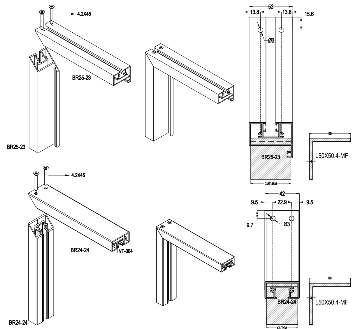
Kombinacija brava + kraća kontra brava za dvokrilna vrata
